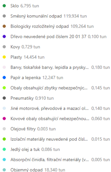
Sumarizační graf
